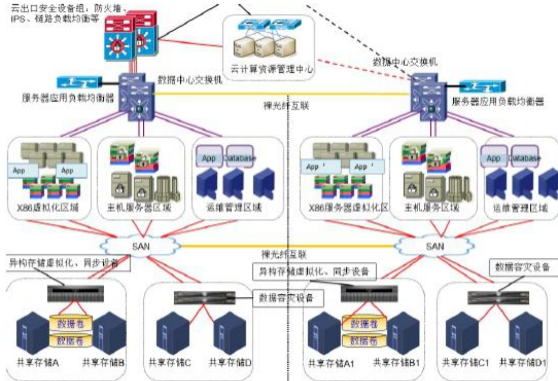
图 3-7 项目云计算服务链接拓扑图
