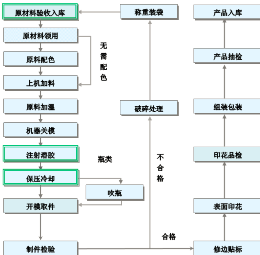
图表 1：注塑（吹塑）工艺流程
